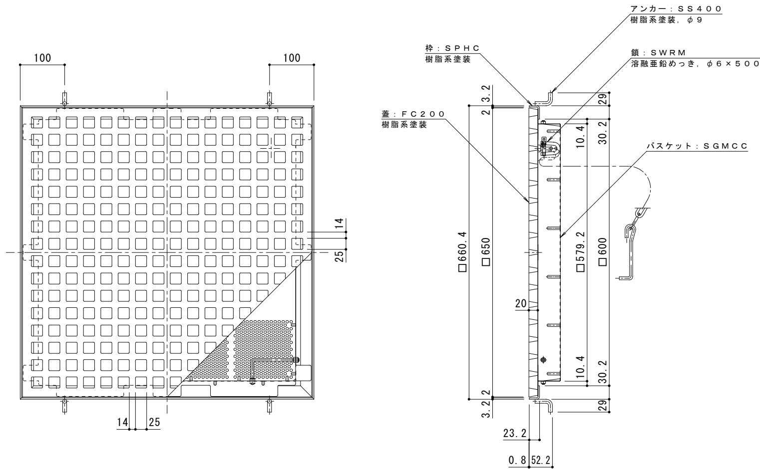
製品詳細図 S = 1 : 6
