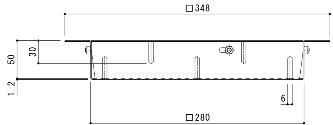
バスケット詳細図 S = 1 : 3
