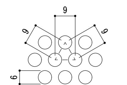
排水穴詳細図 S = 1 : 1
