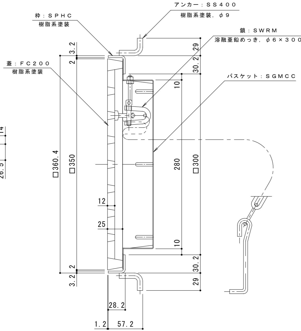
製品詳細図 S = 1 : 3
