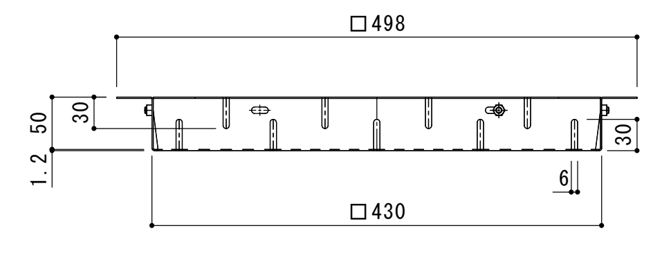
バスケット詳細図 S = 1 : 6
