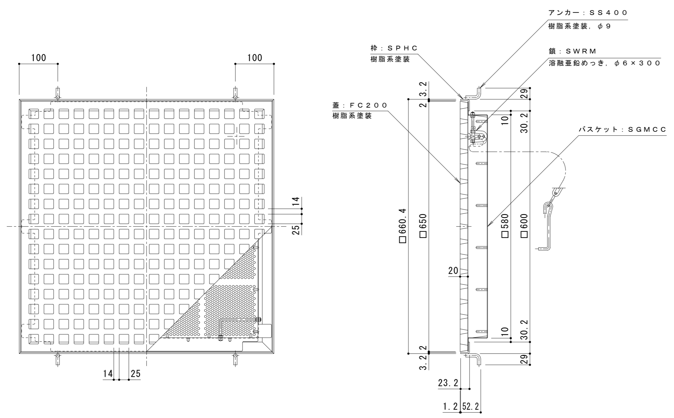
製品詳細図 S = 1 : 6
