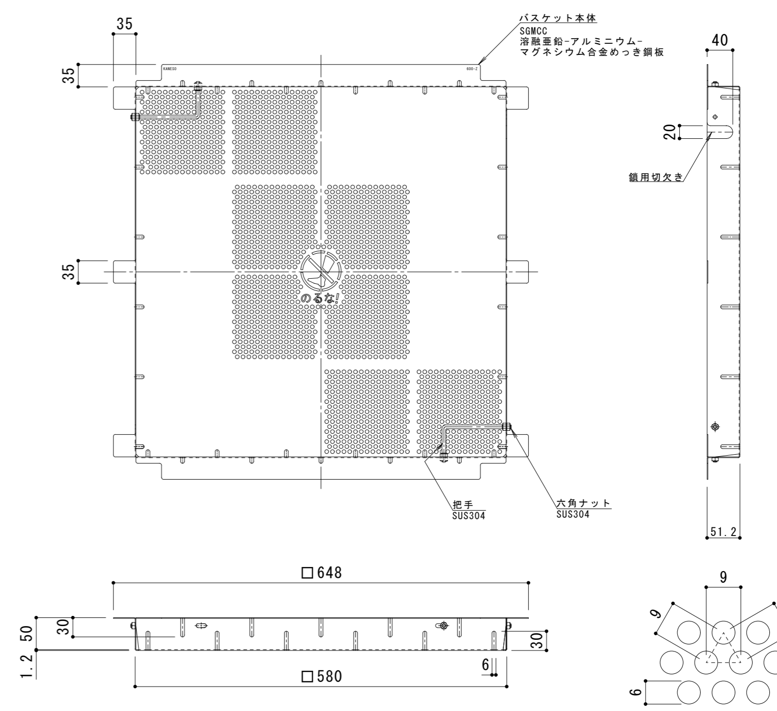
バスケット詳細図 S = 1 : 6
