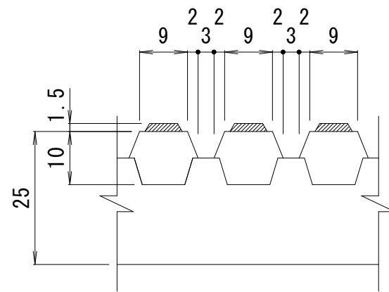
断面詳細図 1:1
