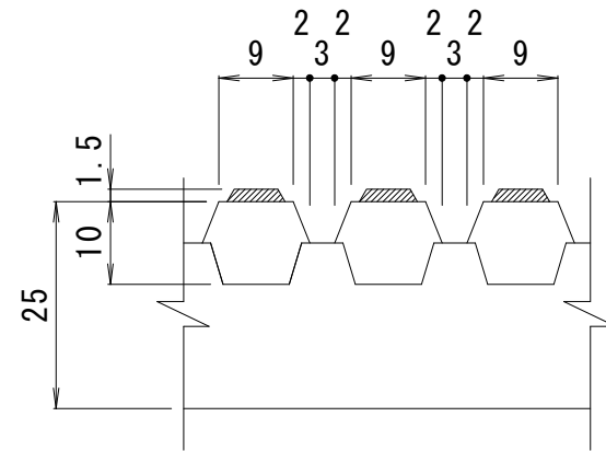
断面詳細図 1:1
