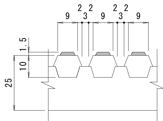
断面詳細図 1:1
