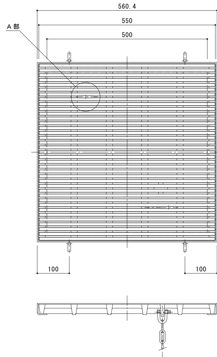
製品詳細図 S = 1 : 5
