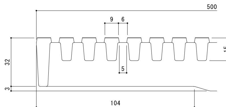
蓋詳細図 S = 1 : 1
