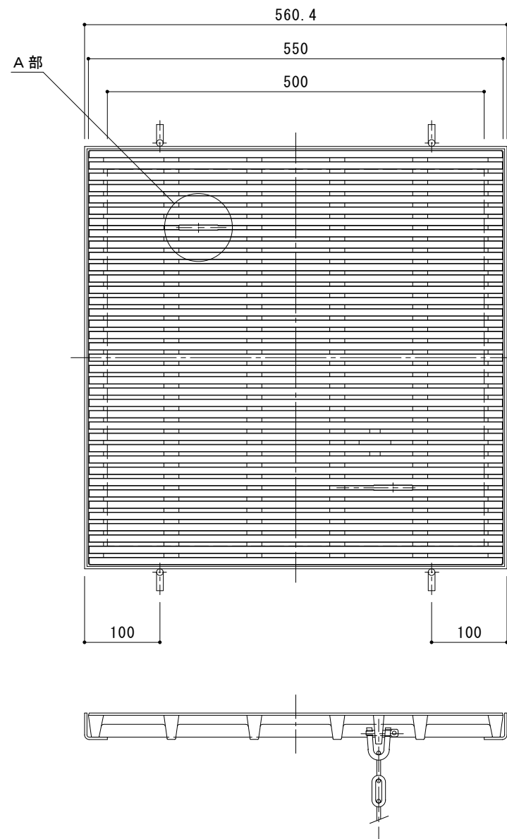
製品詳細図 S = 1 : 5
