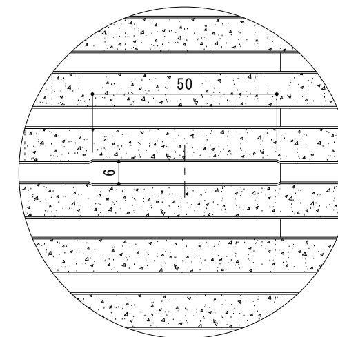
A部 ハンドル差込部詳細図 S = 1 : 1
