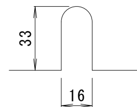
アンカー用切欠部詳細図 S=1:2
