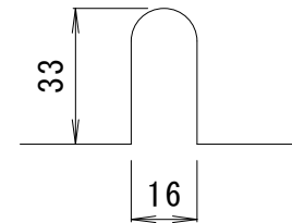
アンカーボルト用切欠部詳細図 S=1:2
