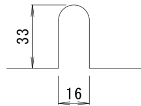
アンカー用切欠部詳細図 S = 1 : 2
