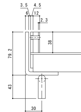
把手部断面詳細図 S=1:2
