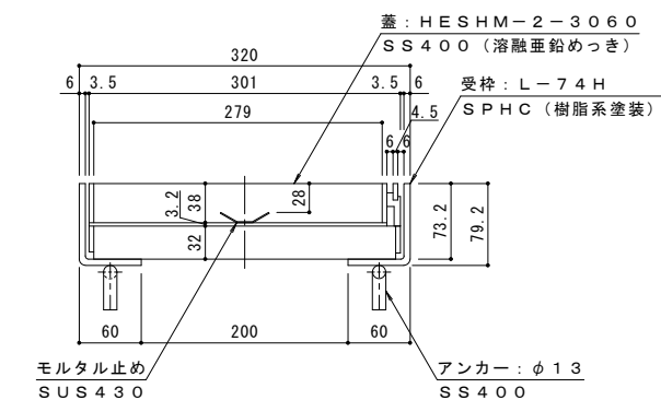
B-B断面図 S=1:4
