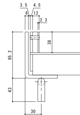
把手部断面詳細図 S=1:2
