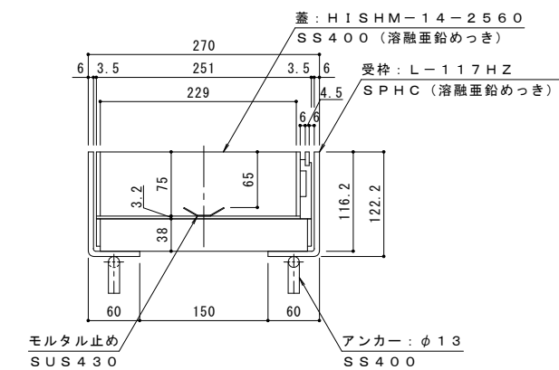
B-B断面図 S = 1 : 4
