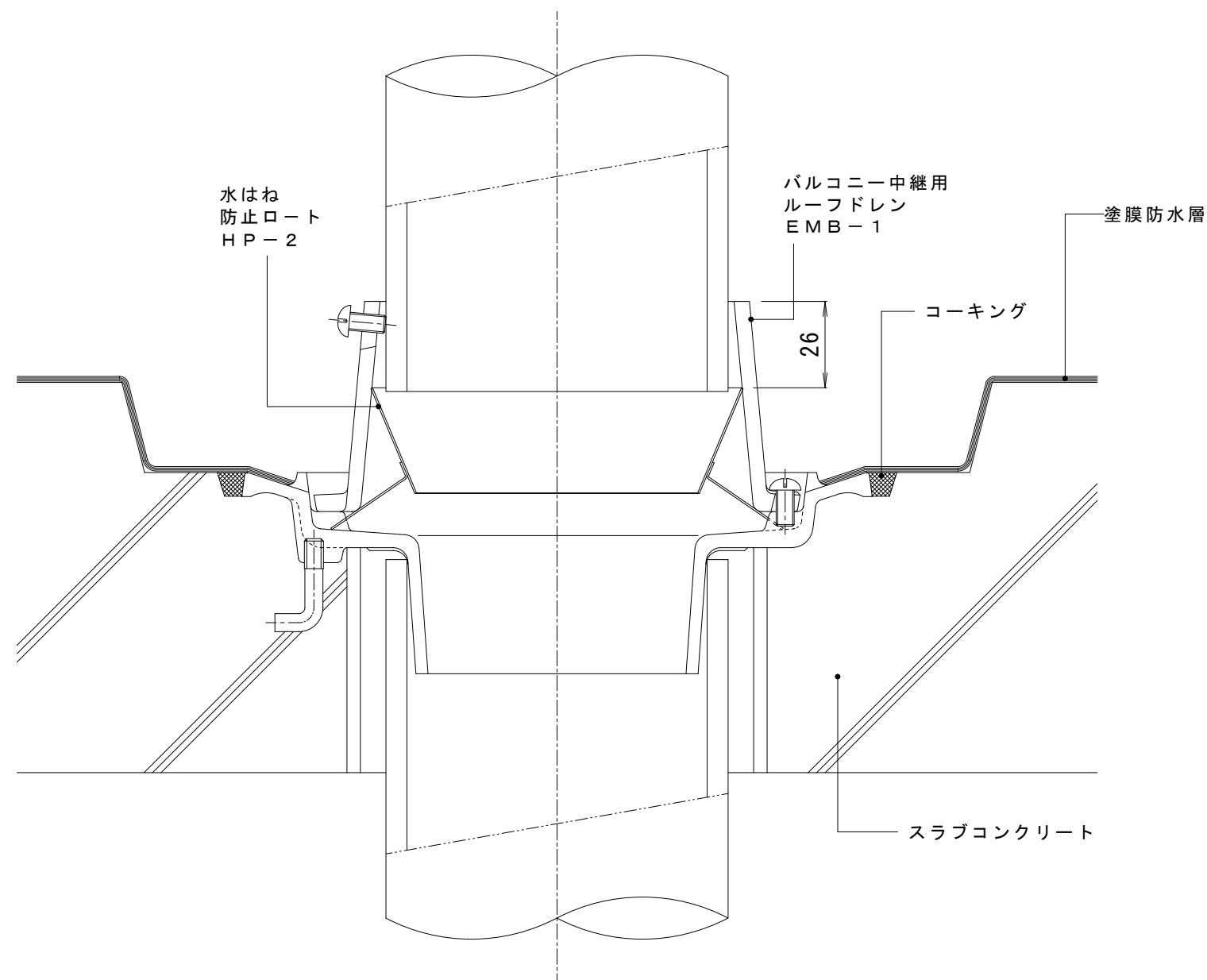
納まり図
