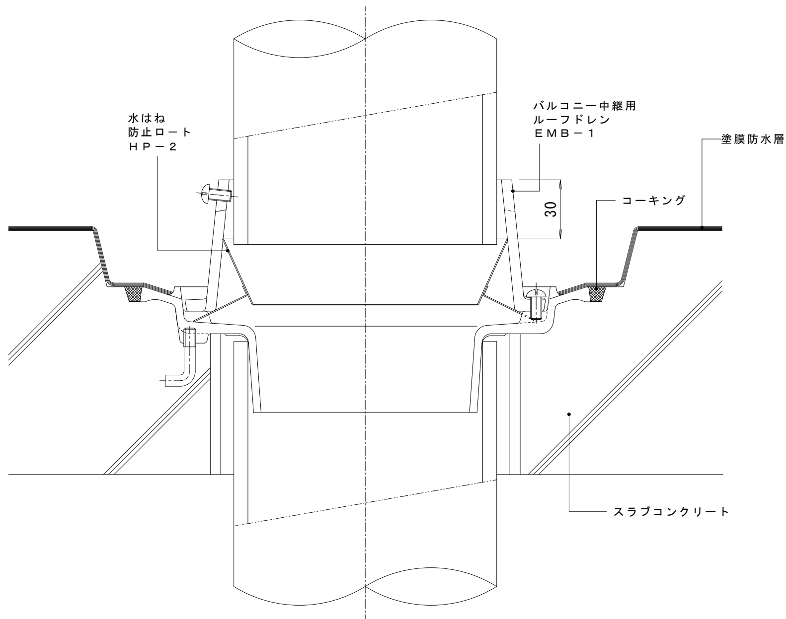
納まり図
