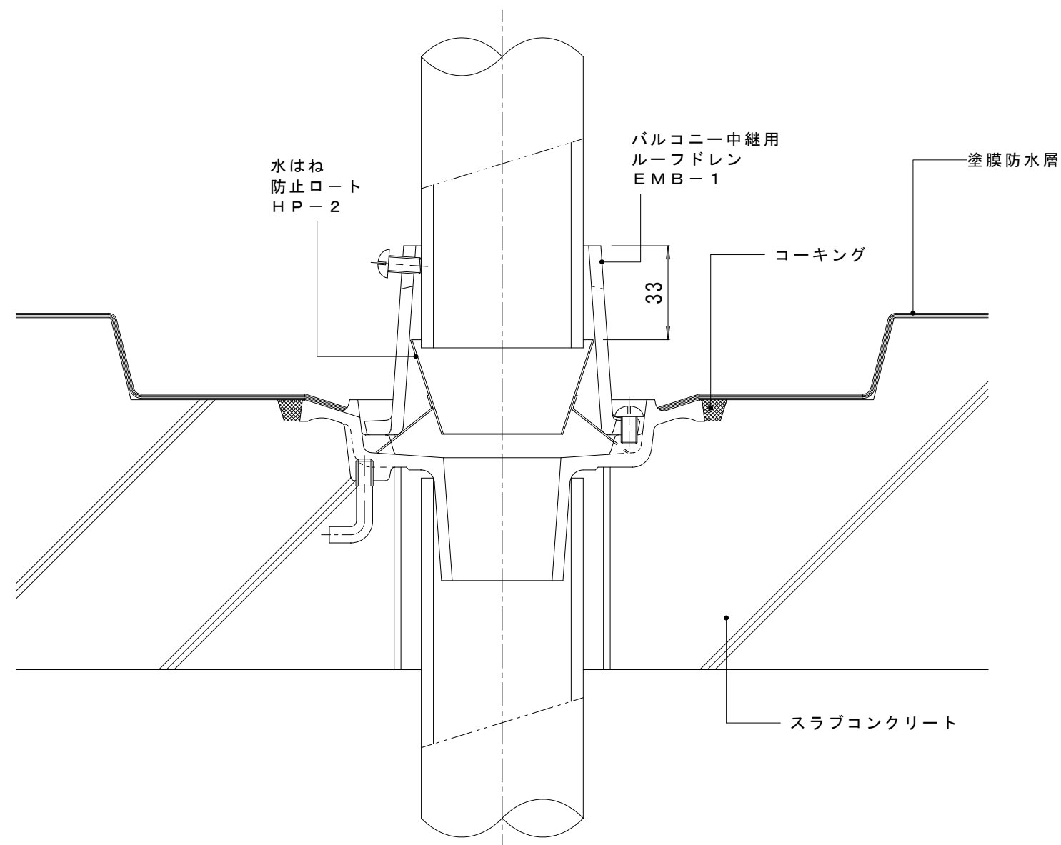
納まり図
