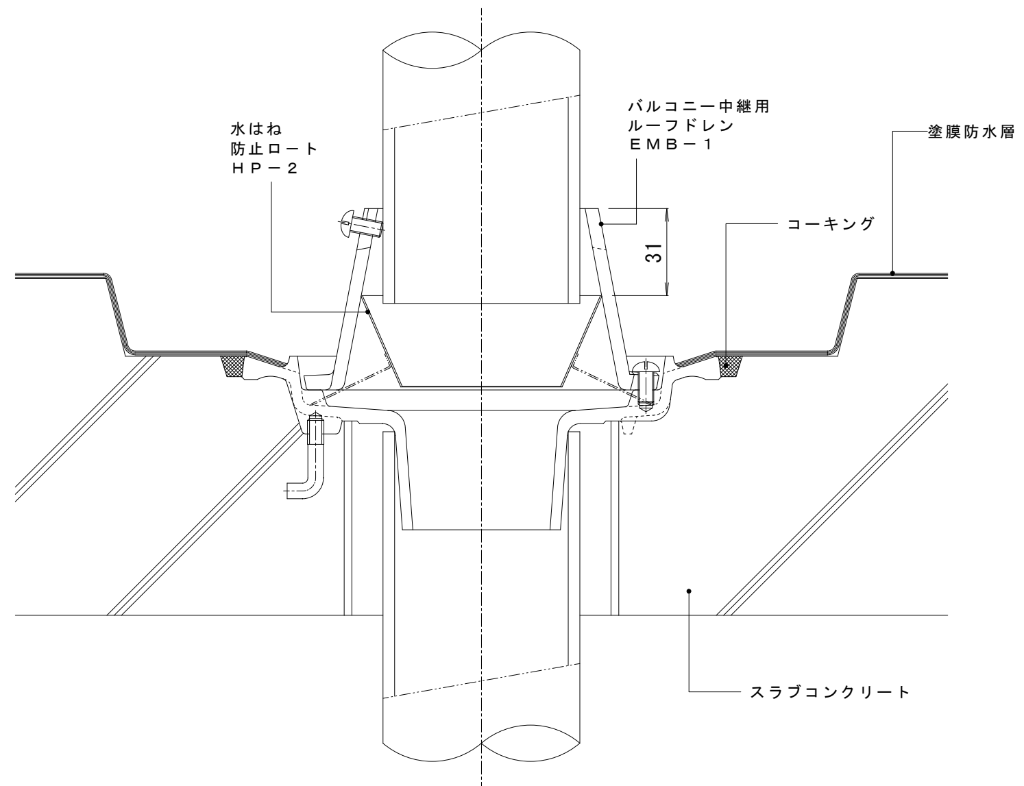
納まり図
