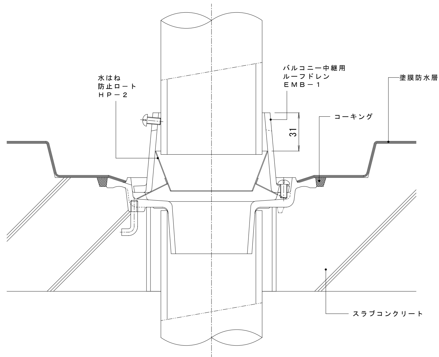
納まり図
