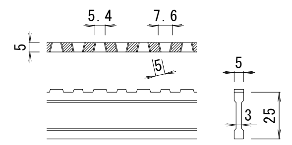
DI-25 バー形状詳細 S=1:2
