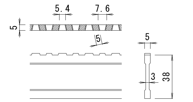
DI-38 バー形状詳細 S=1:2
