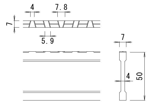
NSI-50 バー形状詳細 S=1:2
