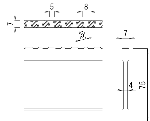
D I - 7 5 バ一形状詳細 S = 1 : 2
