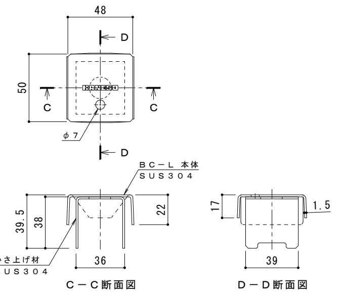
ボルトキャップBC-L詳細図
