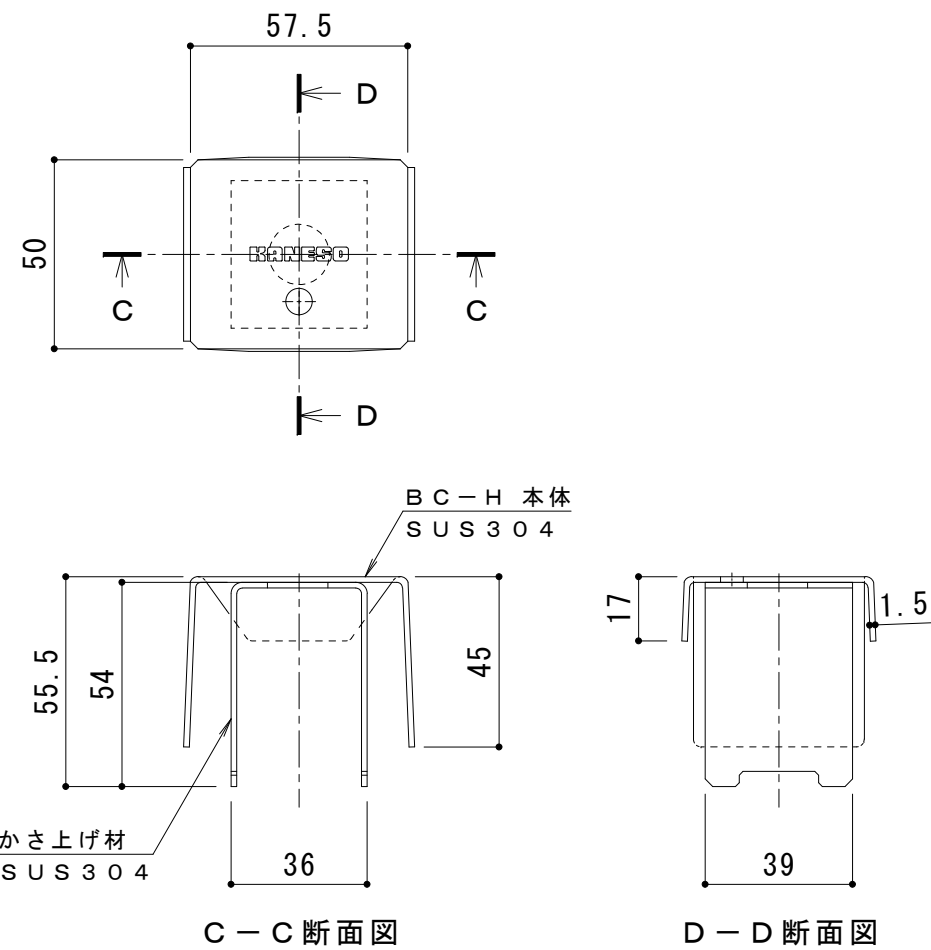
ボルトキャップBC-H詳細図
