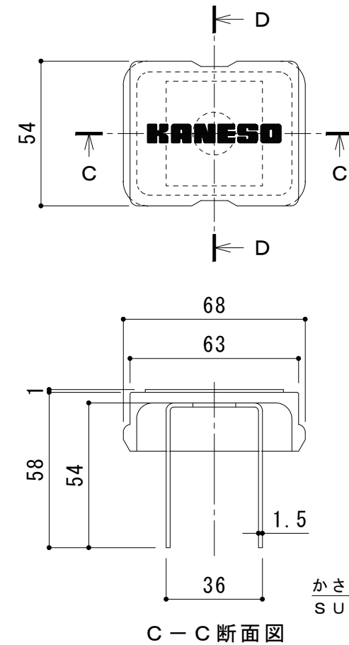
ボルトキャップHC-H詳細図
