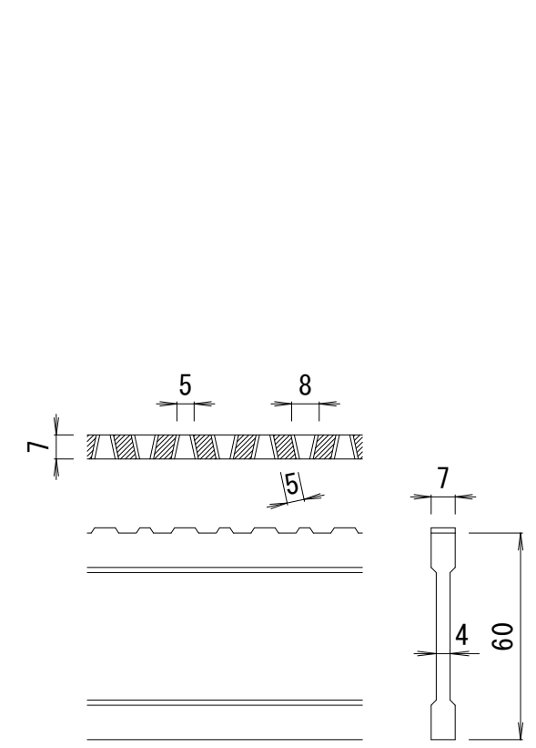
DI-60 バー形状詳細 S = 1 : 2
