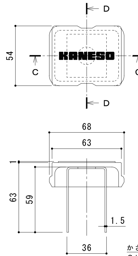
C-C断面図
