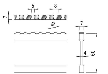
DI-60 バー形状詳細 S = 1 : 2
