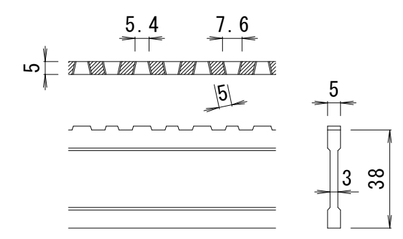
DI-38 バー形状詳細 S=1:2
