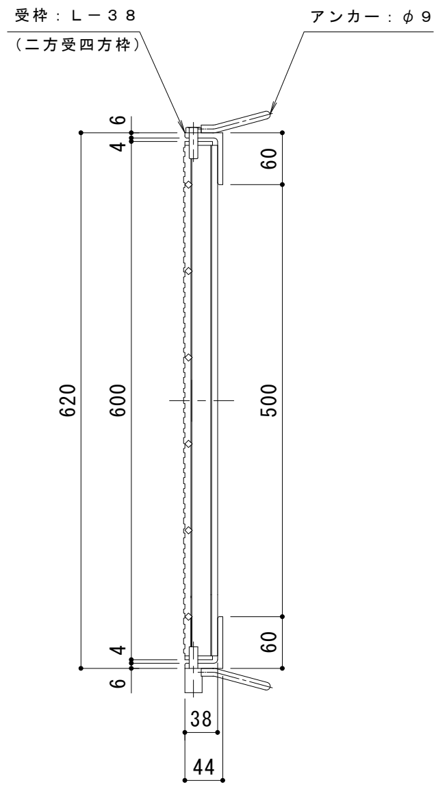
DI-38 バー形状詳細 S=1:2
