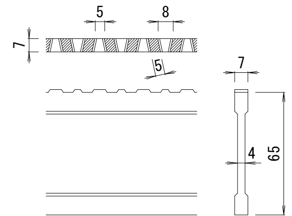
DI-65 バー形状詳細 S=1:2
