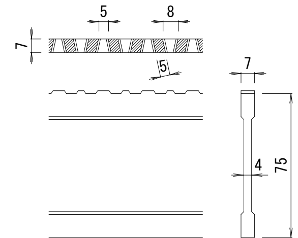
DI-75 バー形状詳細 S=1:2
