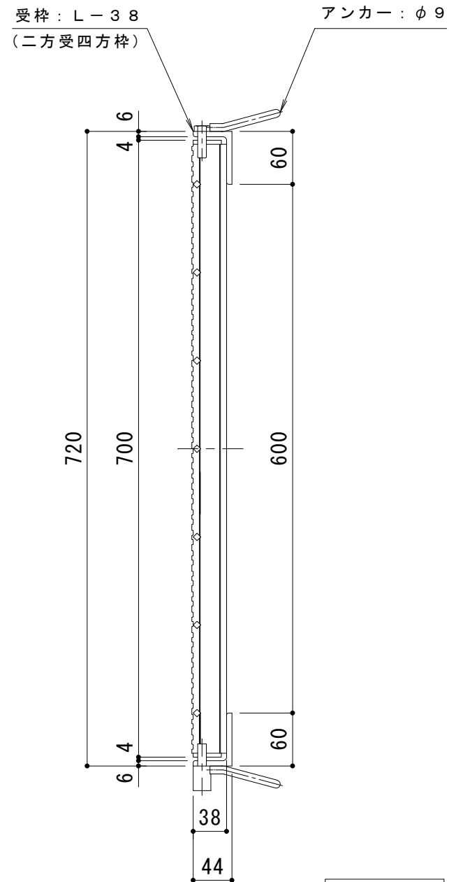
DI-38 バー形状詳細 S=1:2
