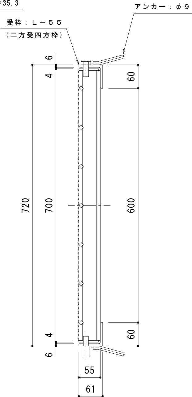
DI-55 バー形状詳細 S=1:2
