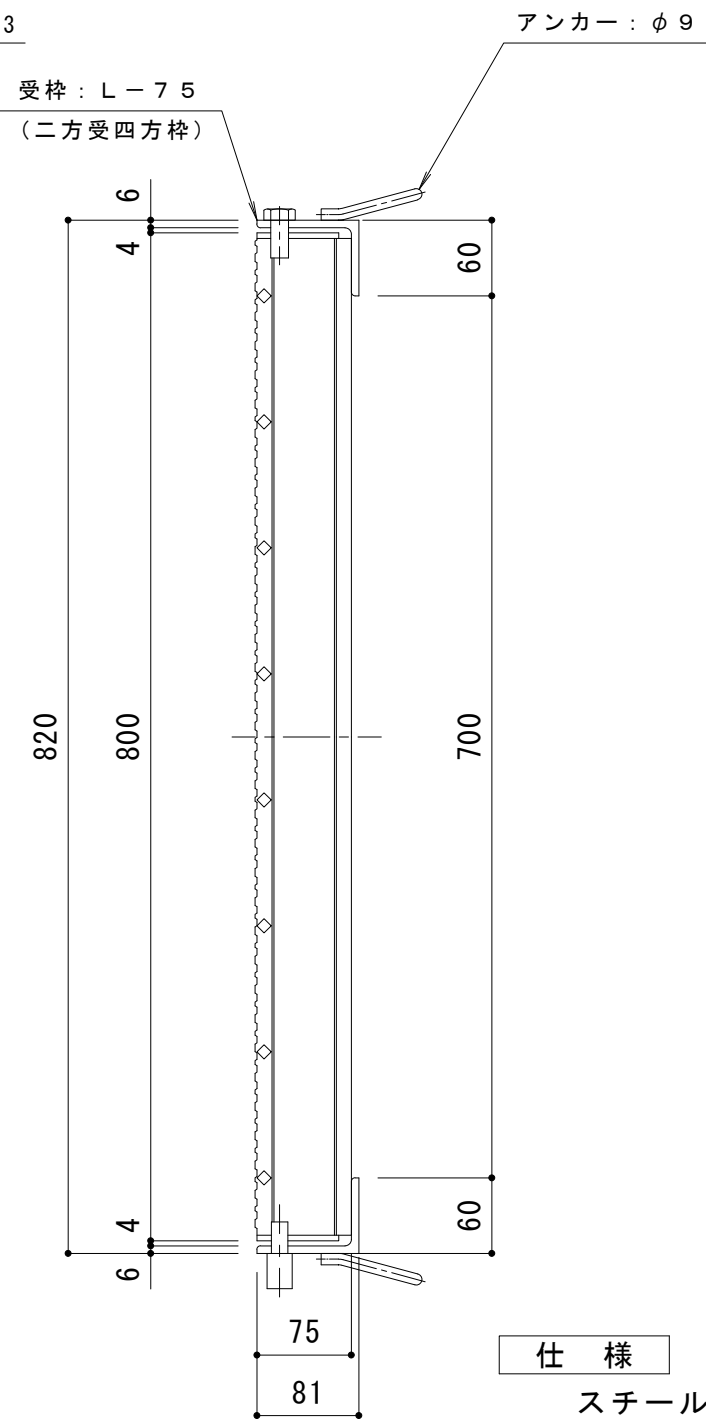
DI-75 バー形状詳細 S=1:2
