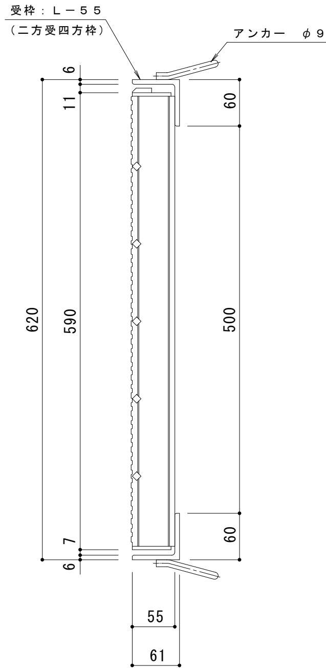
DI-55 バー形状詳細 S=1:2
