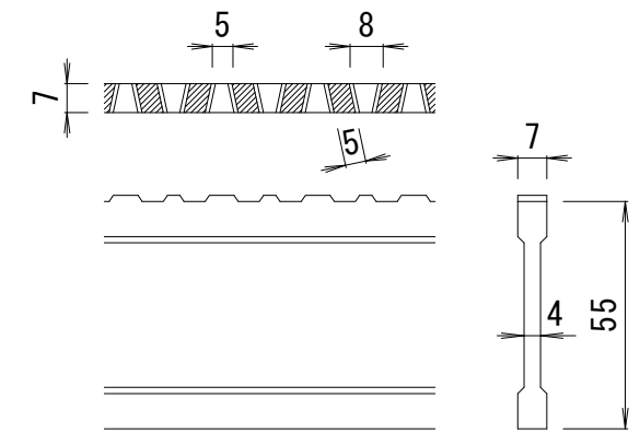
DI-55 バー形状詳細 S=1:2
