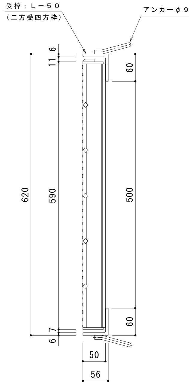
NSI-50 バー形状詳細 S=1:2
