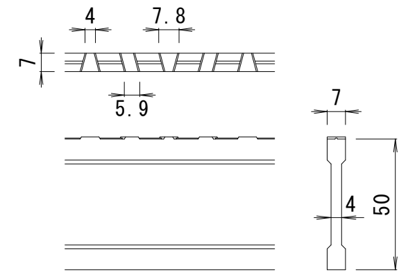
NSI-50 バー形状詳細 S=1:2
