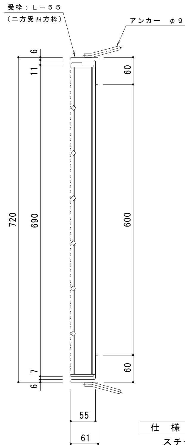
DI-55 バー形状詳細 S=1:2
