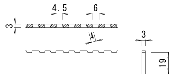
DFB3 x 19 バー形状詳細 S = 1 : 2
