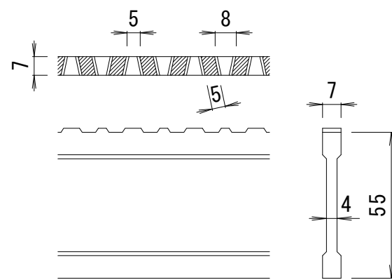
DI-55 バー形状詳細 S=1:2
