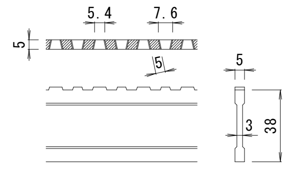
DI-38 バー形状詳細 S=1:2
