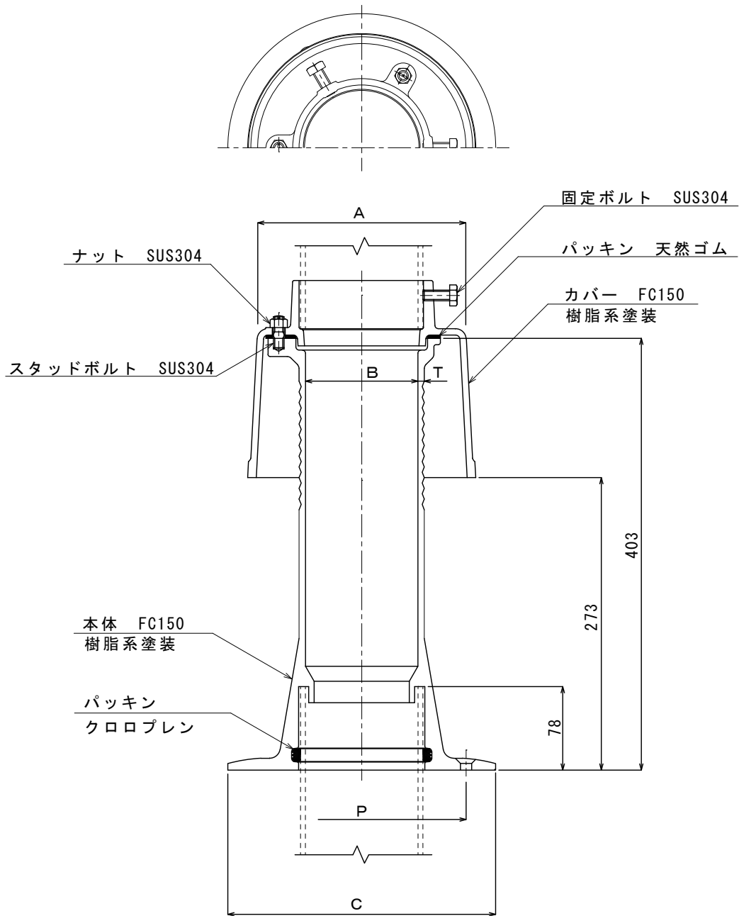
寸法表
