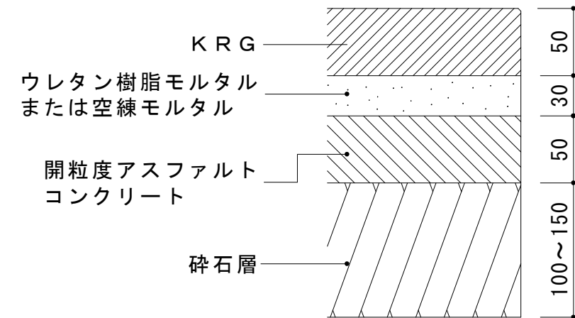
車両乗り入れ部 S = 1 : 4
