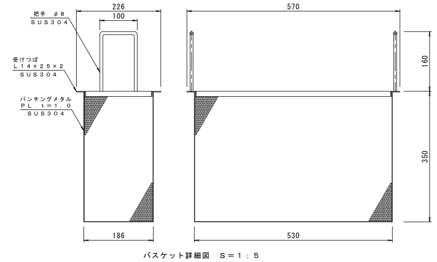
バスケット詳細図 S=1:5
