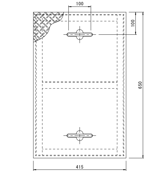
蓋詳細図 S=1:5 表面処理: エポキシ樹脂コーティング (色: グレー)
