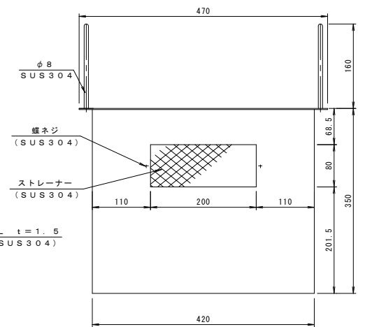
バスケット詳細図 S=1:5
