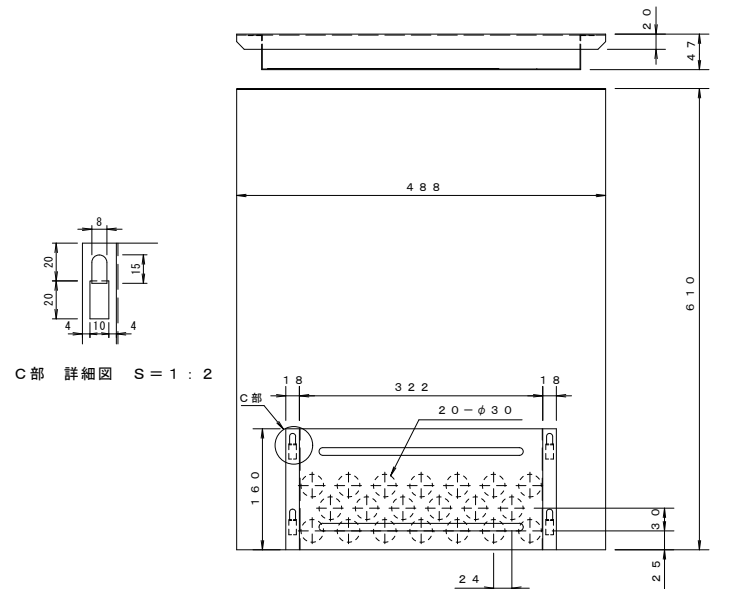
可動式隔板詳細図 S=1:5
