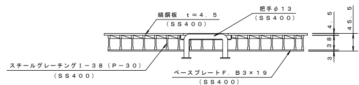
蓋詳細図 S=1:5 表面処理: 溶融亜鉛メッキ
