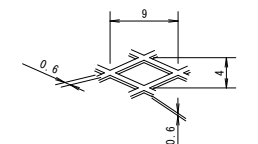
バスケット網詳細図 S=2:1
