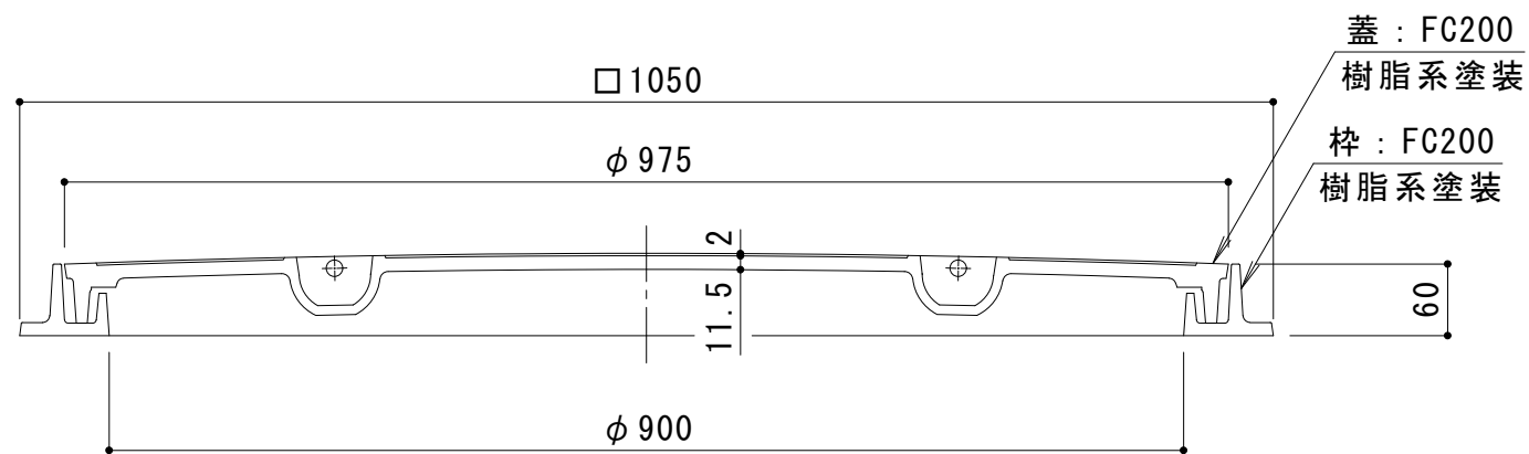
A-A断面図
