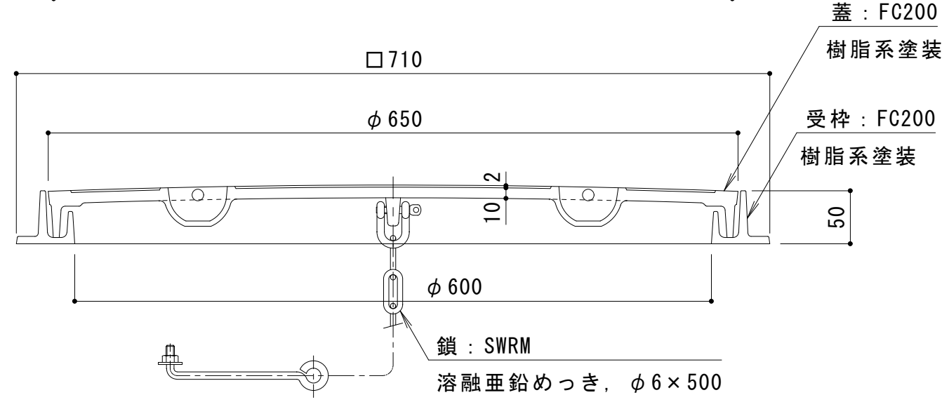
A-A 断面図
