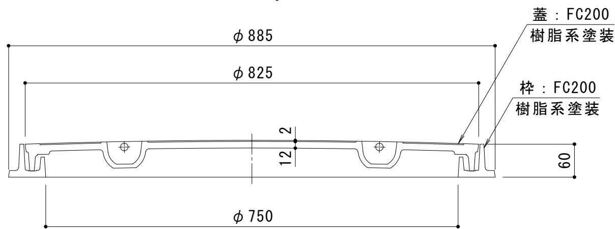
A-A断面図
